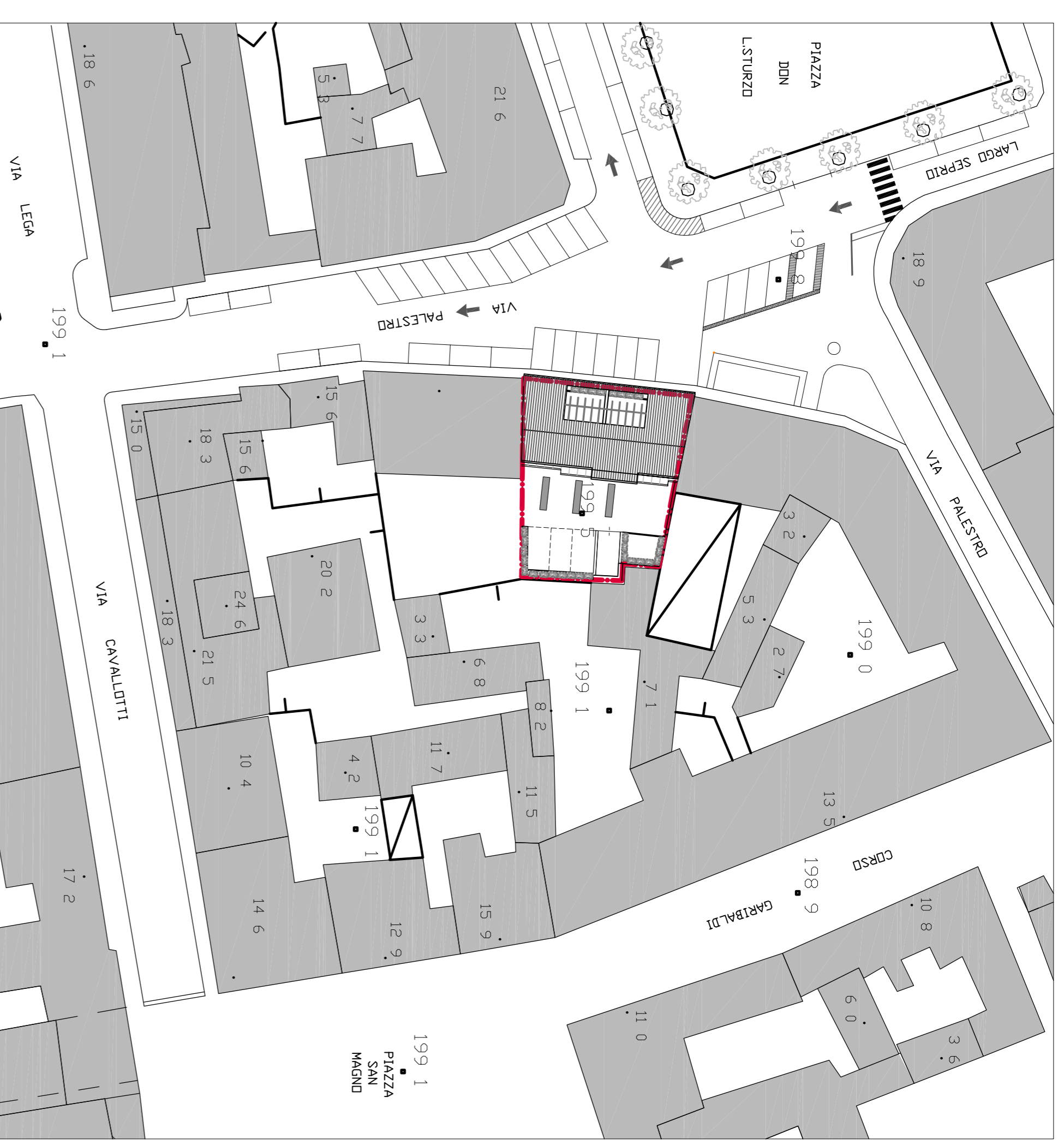
PLANIMETRIA scala 1:500
