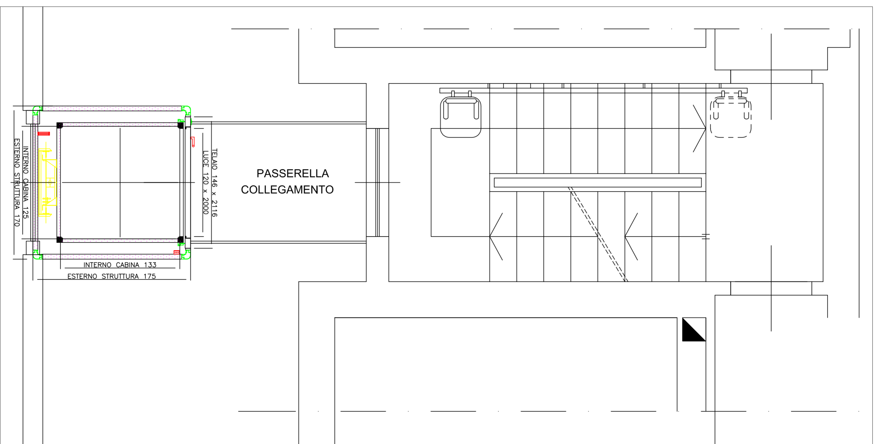
PARTICOLARE POSIZIONAMENTO ASCENSORE E SERVOSCALA
