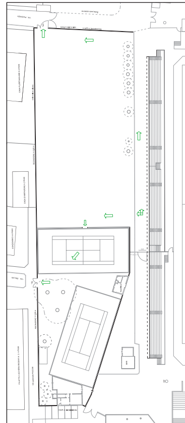
PLANIMETRIA GENERALE DELLO STATO DI FATTO SCALA 1: 500
