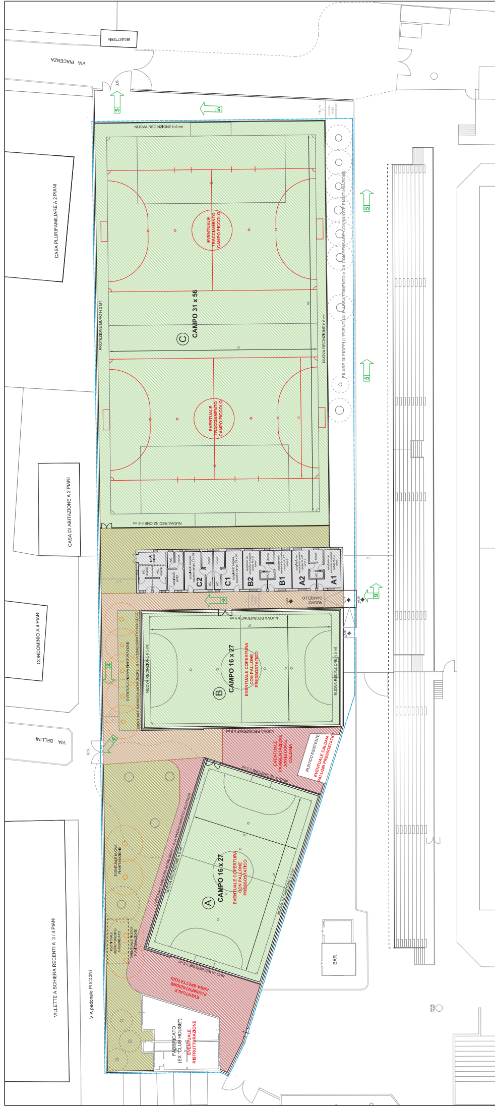
PLANIMETRIA GENERALE DI PROGETTO SCALA 1: 200
